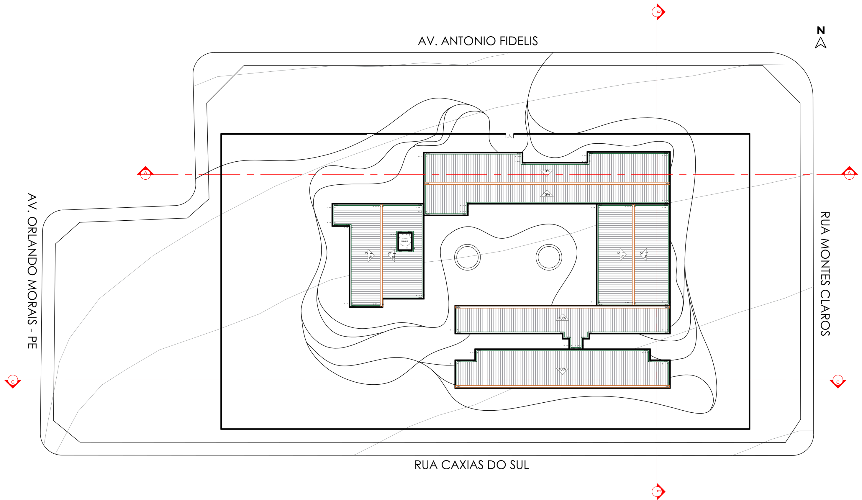
5 PLANTA DE COBERTURA ESCALA: 1:500
