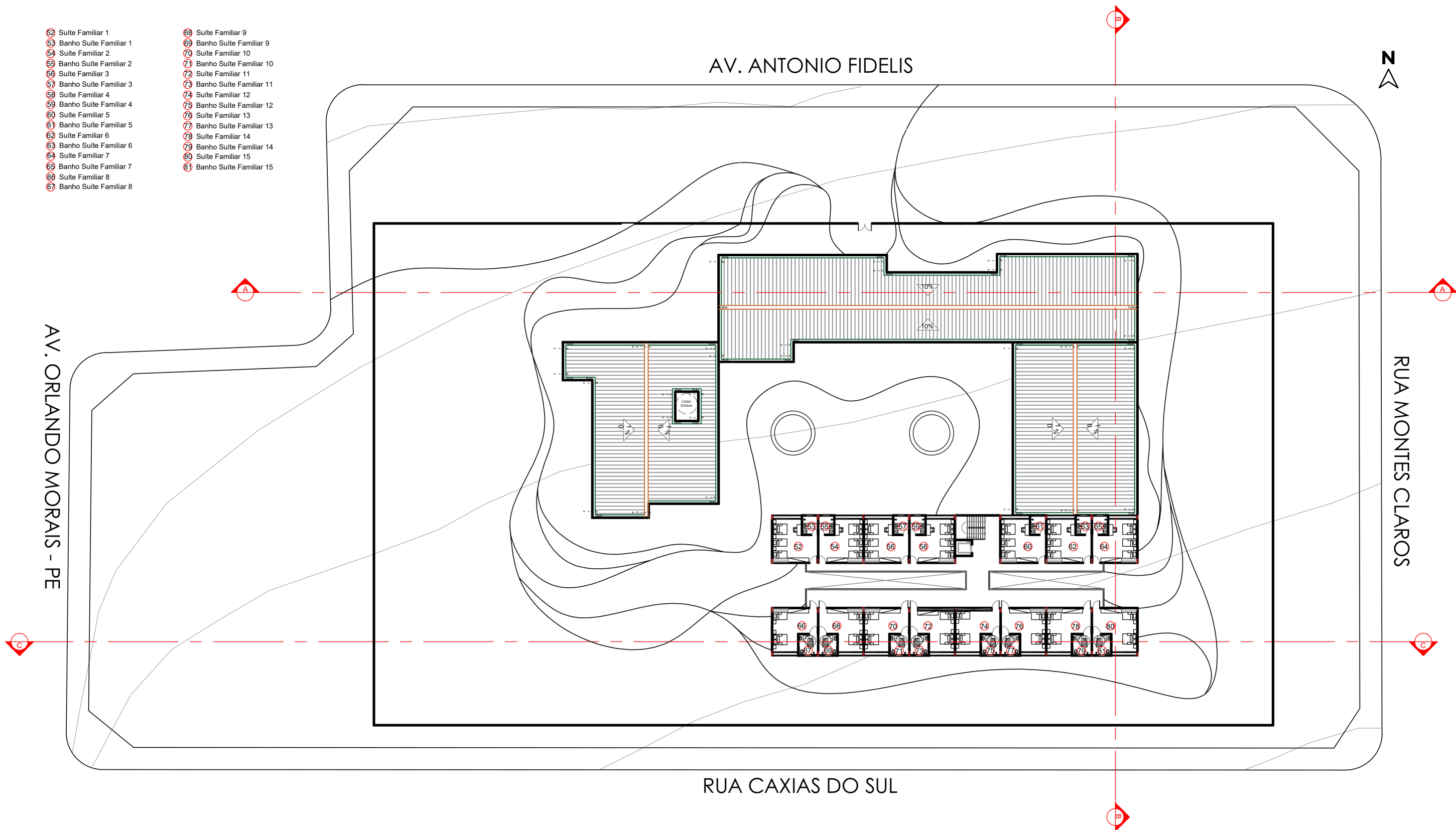
3 PLANTA DO PAVIMENTO SUPERIOR 1 ESCALA: 1:500
