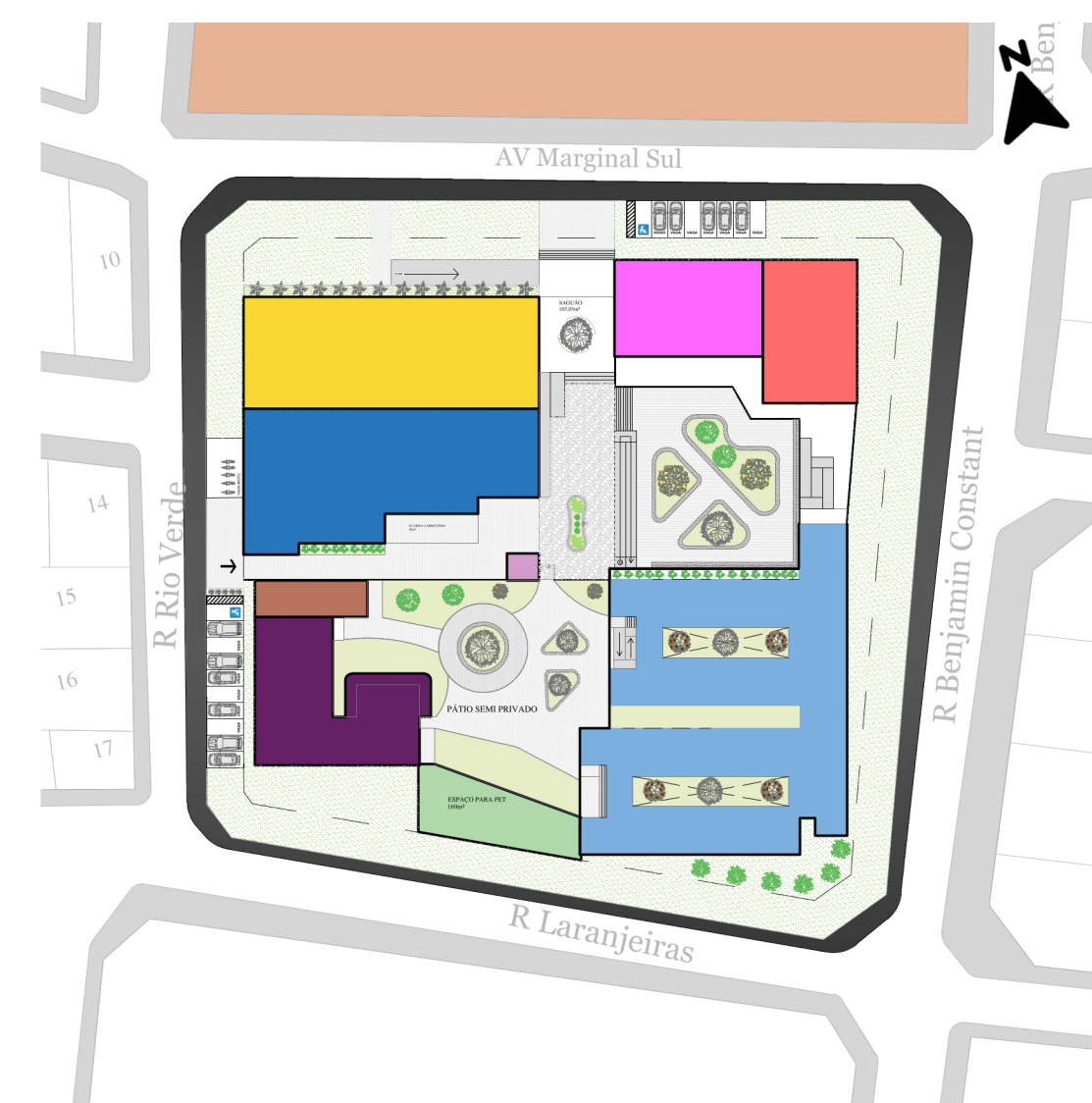
18 Setorização Esc 1:500
