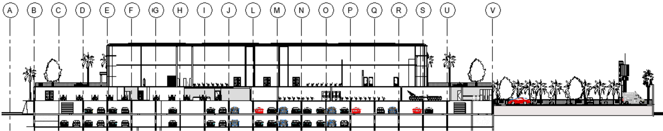
CORTE (A-A)
