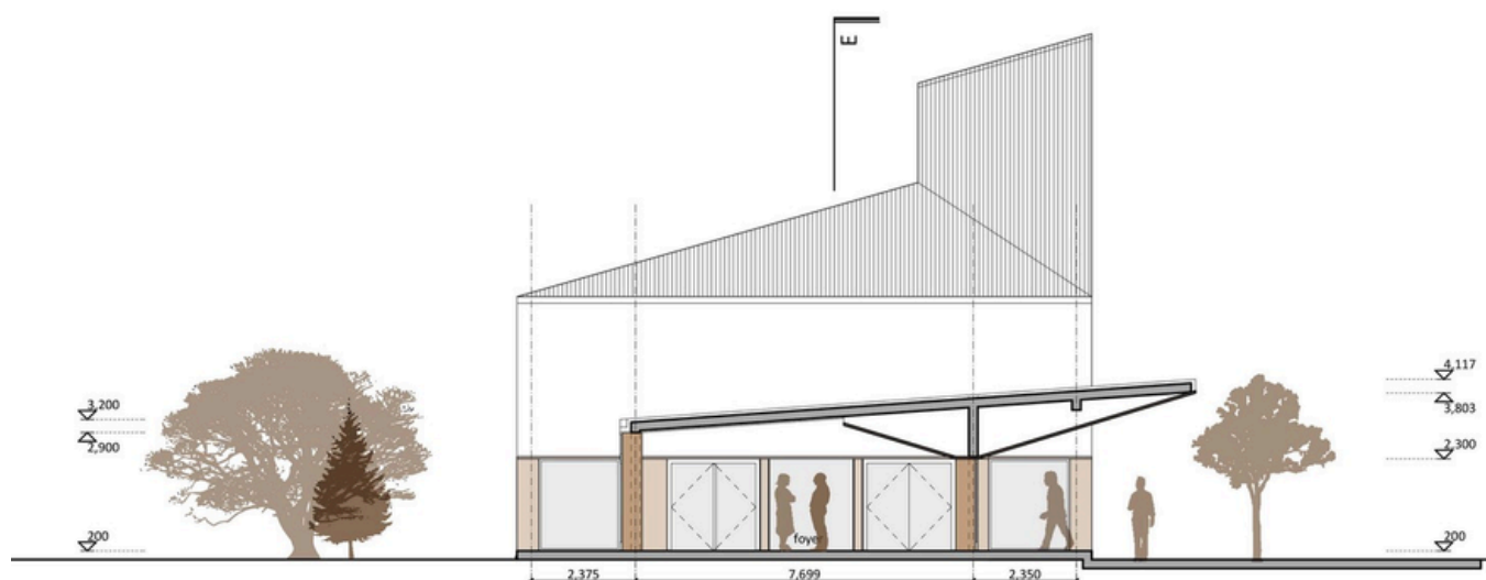
CORTE (A-A) DA IGREJA METODISTA DO NORTE EM CHRISTCHURCH – FONTE: STEPHEN GOODENOUGH
