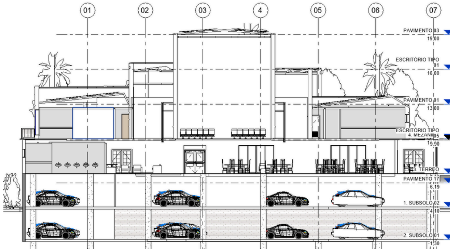
CORTE (D-D)
