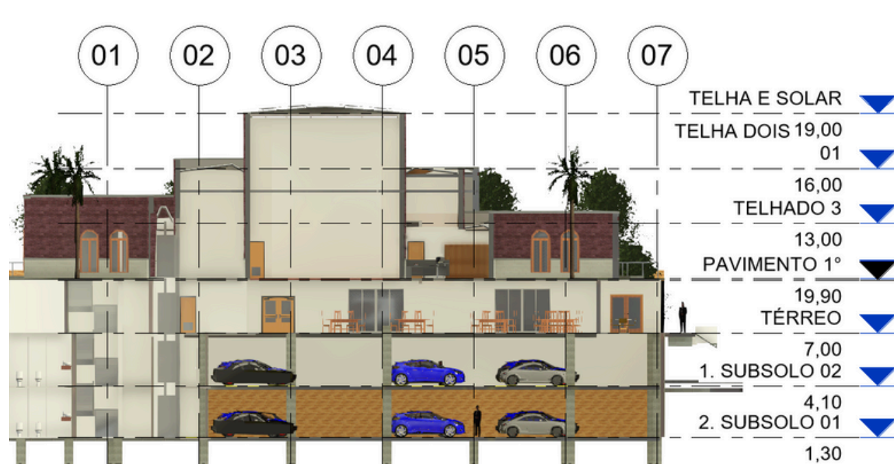
CORTE (B-B)
