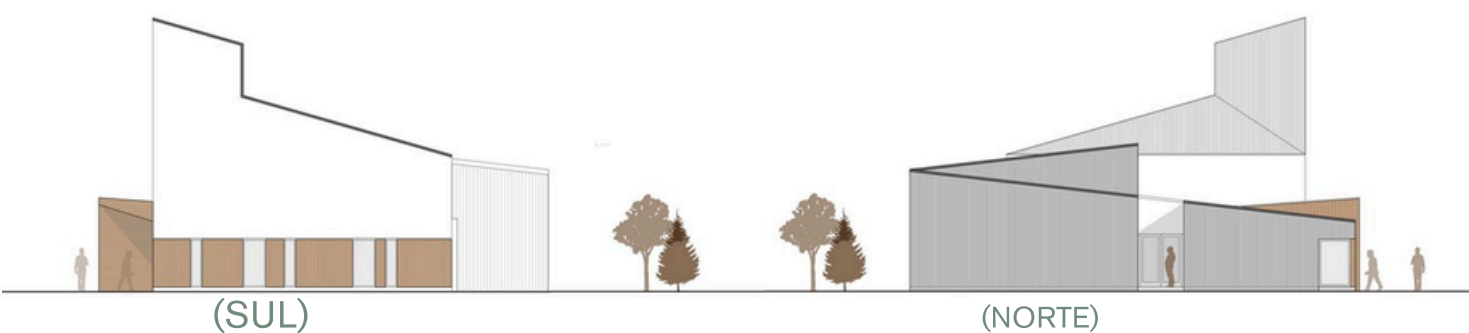
FACHADAS (SUL E NORTE) DA IGREJA METODISTA DO NORTE EM CHRISTCHURCH - FONTE: STEPHEN GOODENOUGH
