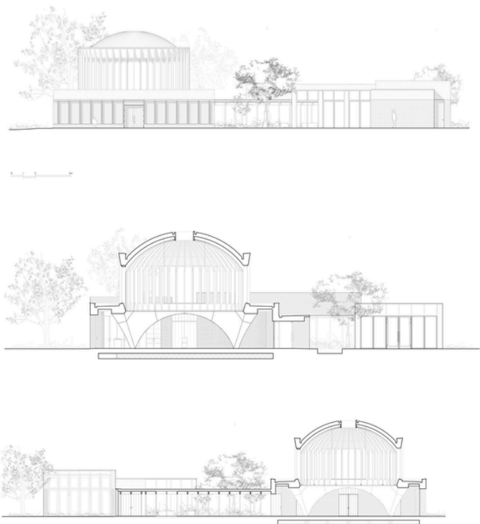
IMAGEM: CORTES- COMPLEXO DO TEMPLO - FONTE: STEPHEN GOODENOUGH
