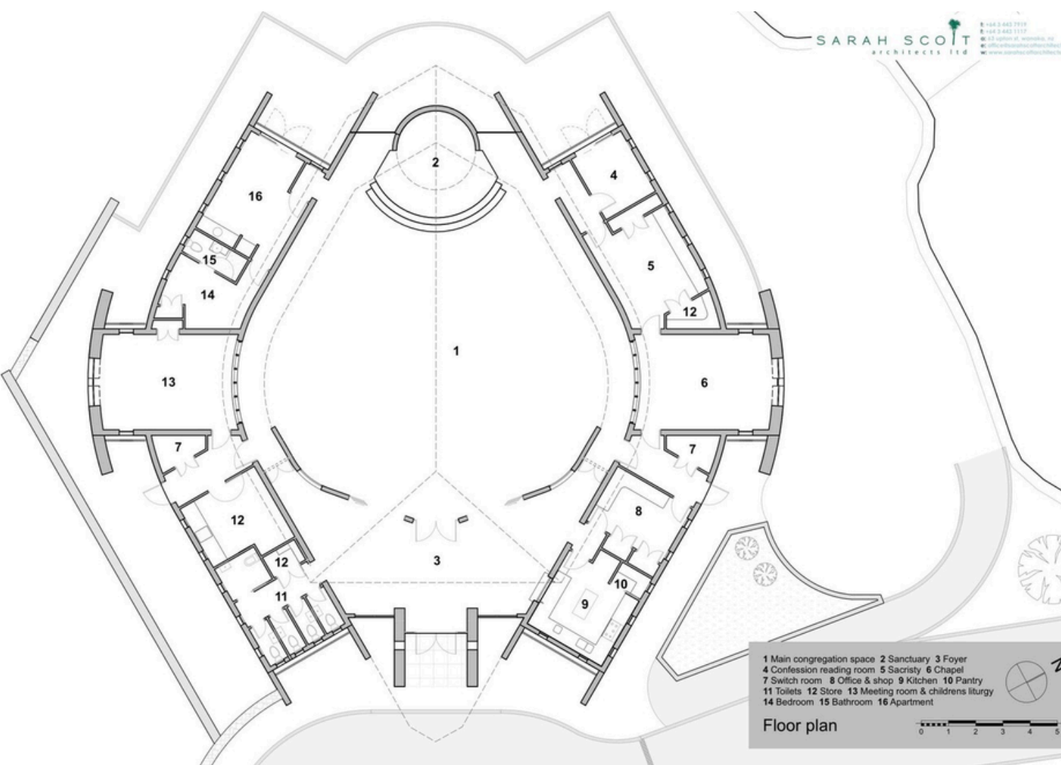
PLANTA BAIXA- IGREJA CATÓLICA DE WANAKA
