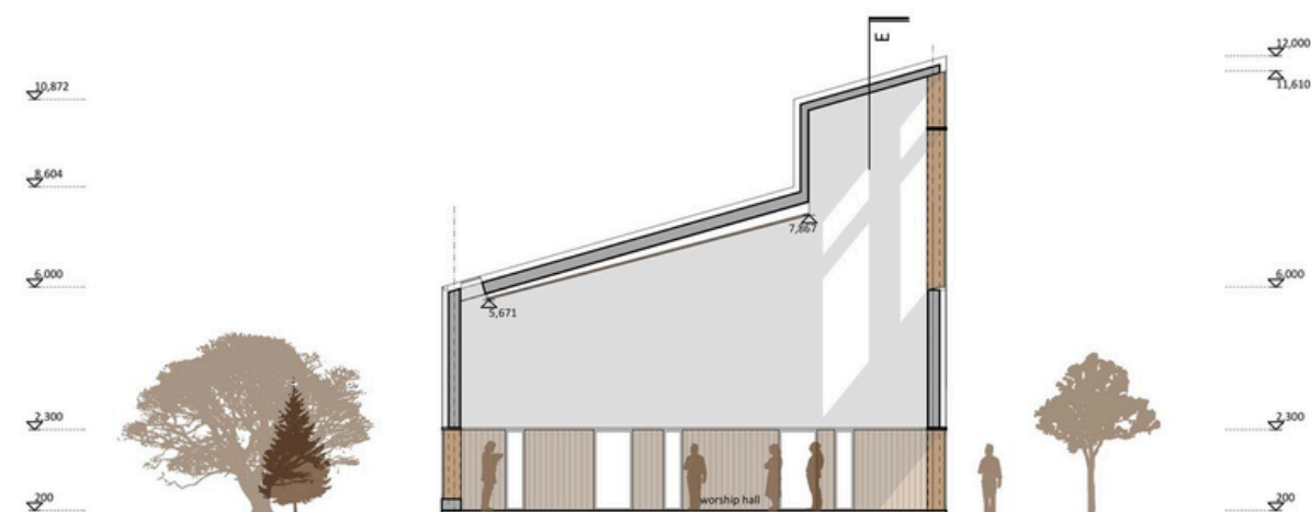
CORTE (B-B) DA IGREJA METODISTA DO NORTE EM CHRISTCHURCH – FONTE: STEPHEN GOODENOUGH
