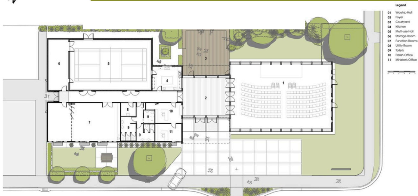
PLANTA BAIXA DA IGREJA METODISTA DO NORTE EM CHRISTCHURCH
