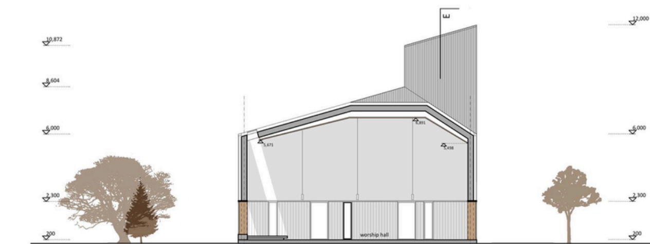
I CORTE (C-C) DA IGREJA METODISTA DO NORTE EM CHRISTCHURCH – FONTE: STEPHEN GOODENOUGH
