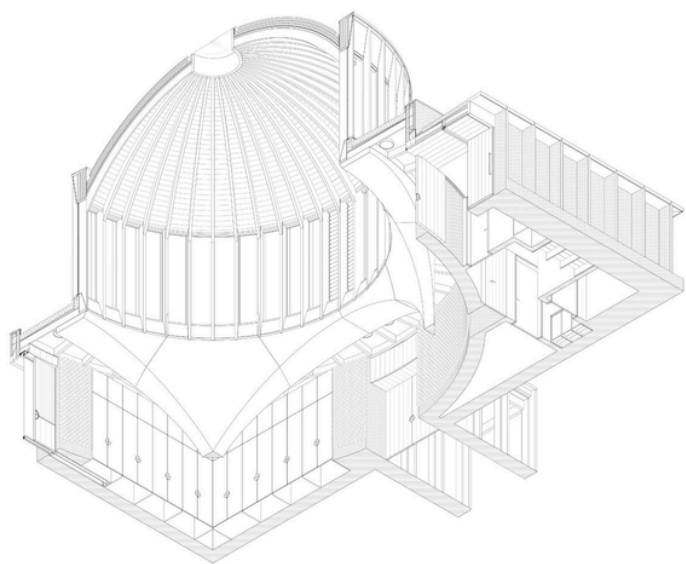
IMAGEM: CORTE - COMPLEXO DO TEMPLO - FONTE: STEPHEN GOODENOUGH
