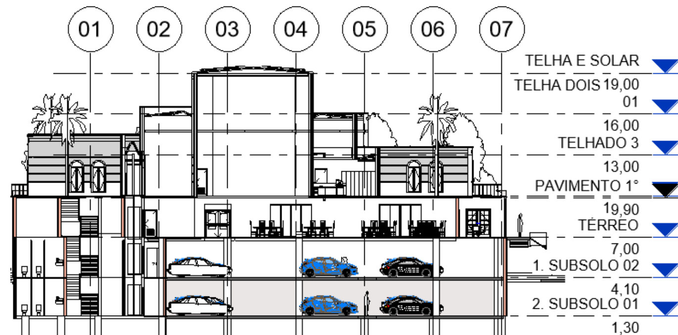
CORTE (B-B)
