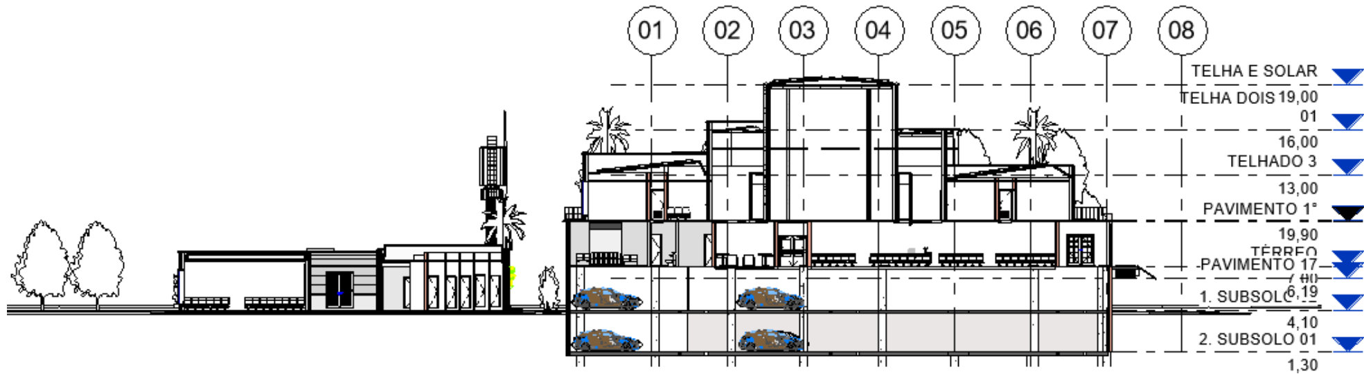
CORTE (B-B)
