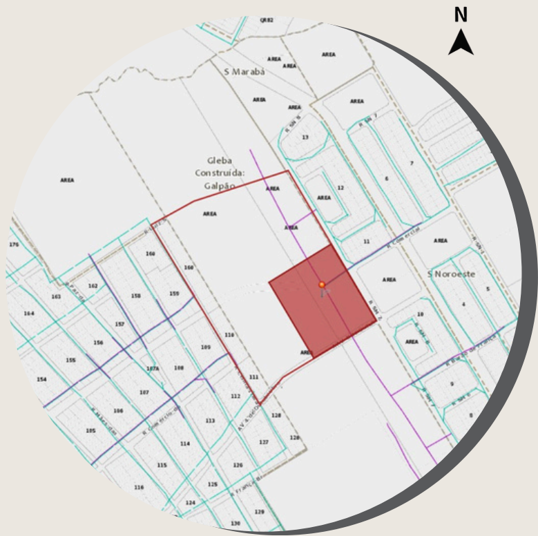
Mapa de Rede Elétrica
