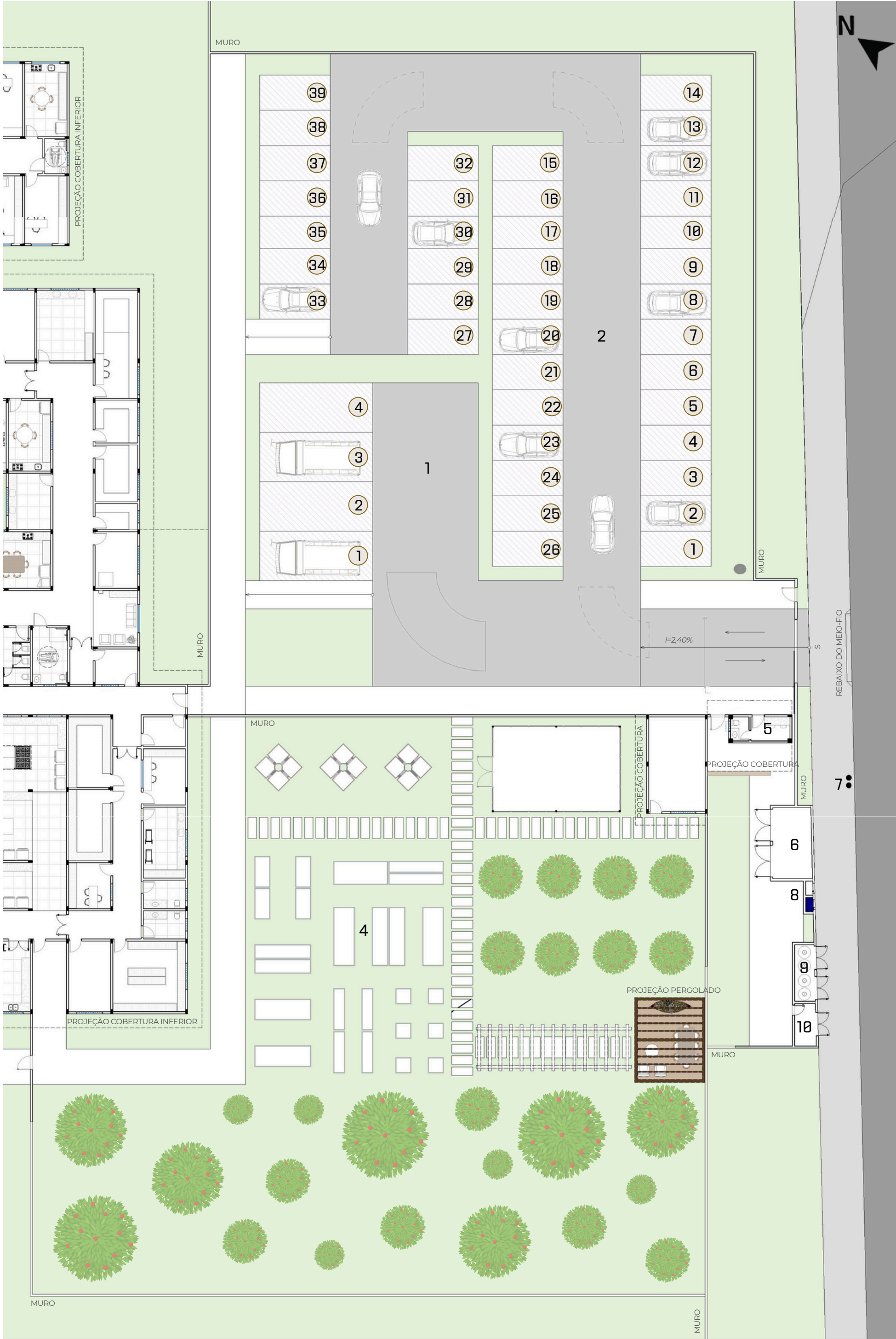
PLANTA ESTACIONAMENTO SERVIÇOS 0 5 10m
