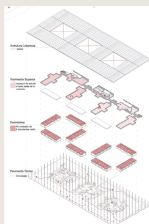
Figura 36: Detalhamento dos pavimentos Fonte: https://www.archdaily.com.br/br/985951/moradias-infantis-em-canua-na-encontro-entre-arquitetura-vernacular-e-tecnologias-industriais
