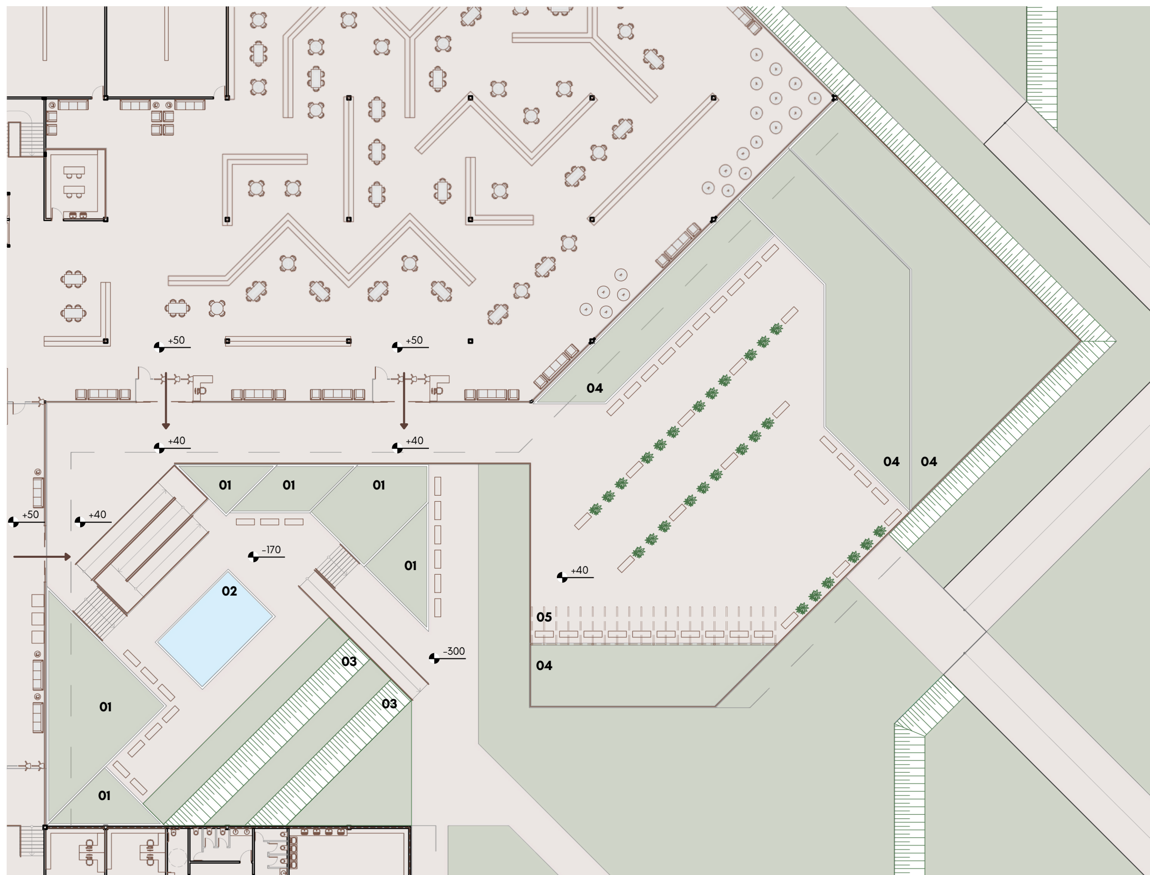
PLANTA DO PÁTIO CENTRAL E TERRAÇO 1 0 1 5m
