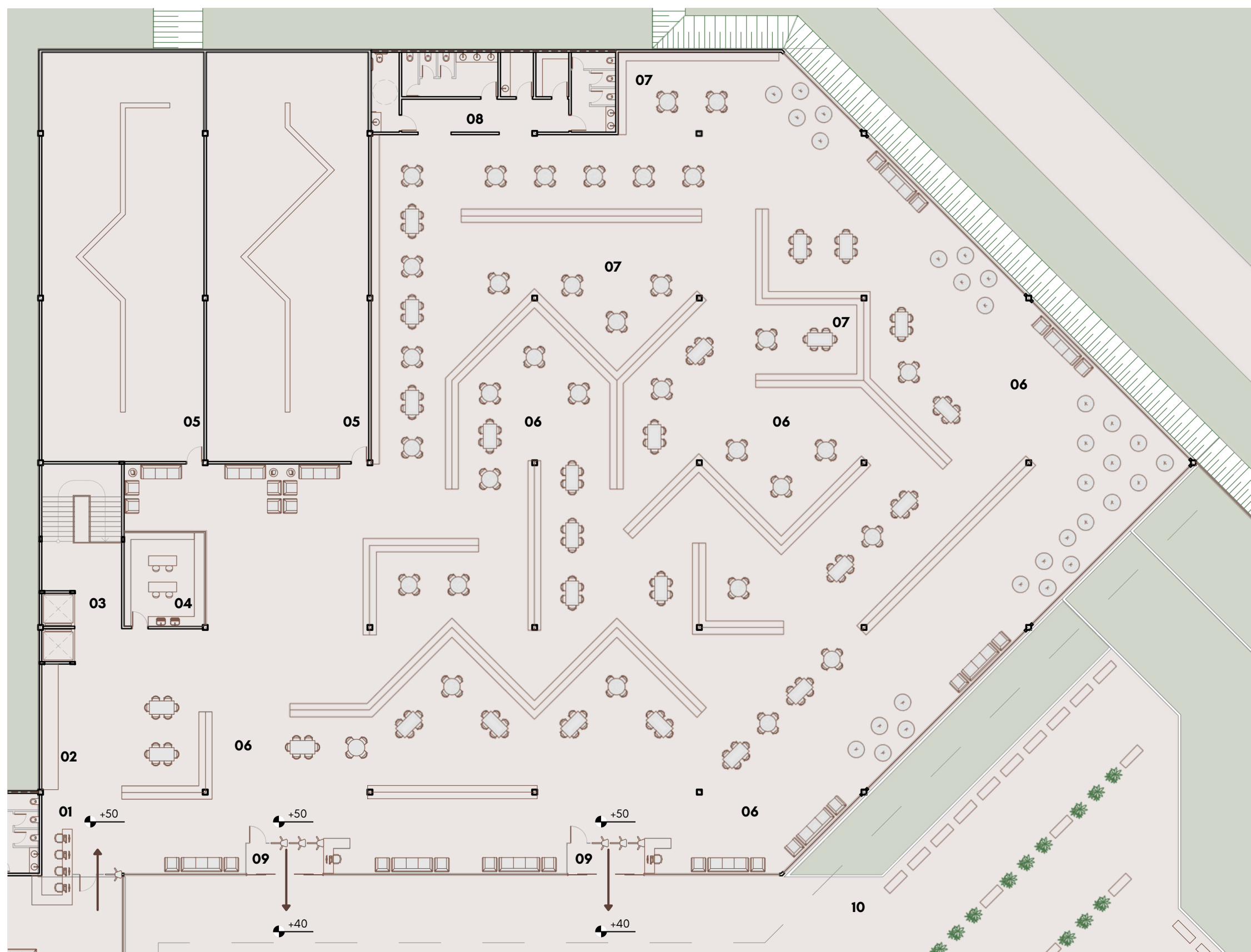
N PLANTA DO SETOR DE ESTUDO E PESQUISA 0 1 5m
