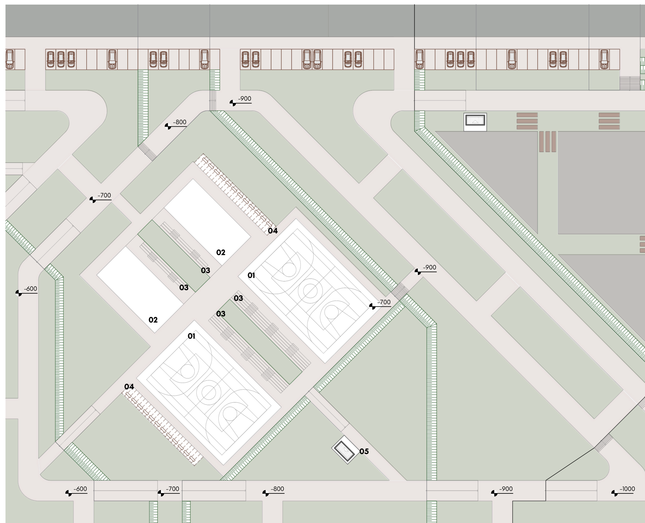
PLANTA DO SETOR DE ESPORTES COLETIVOS
