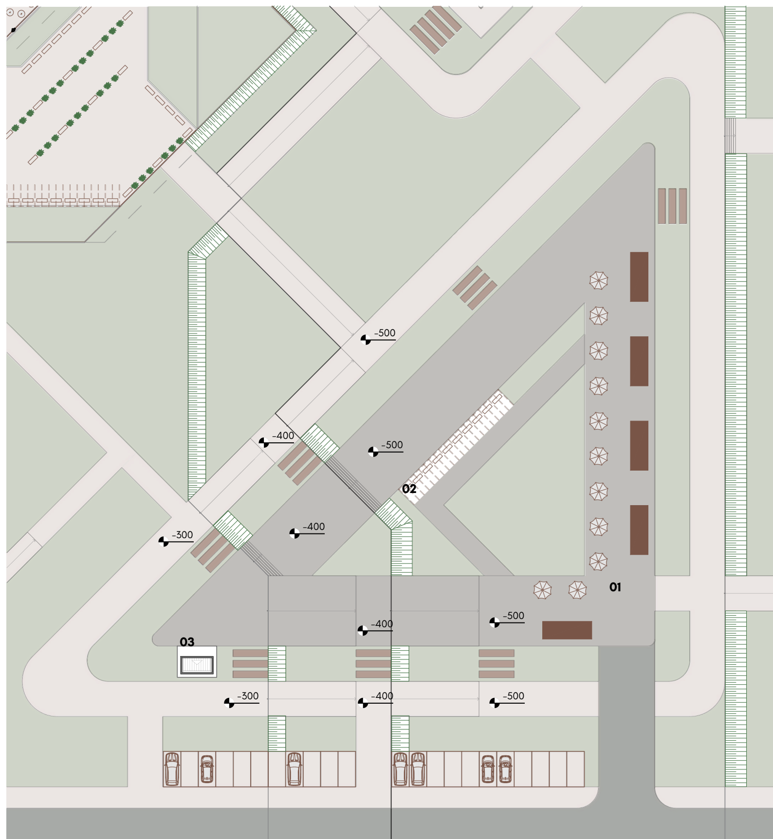
PLANTA DO SETOR GASTRONÔMICO 01 5 10m
