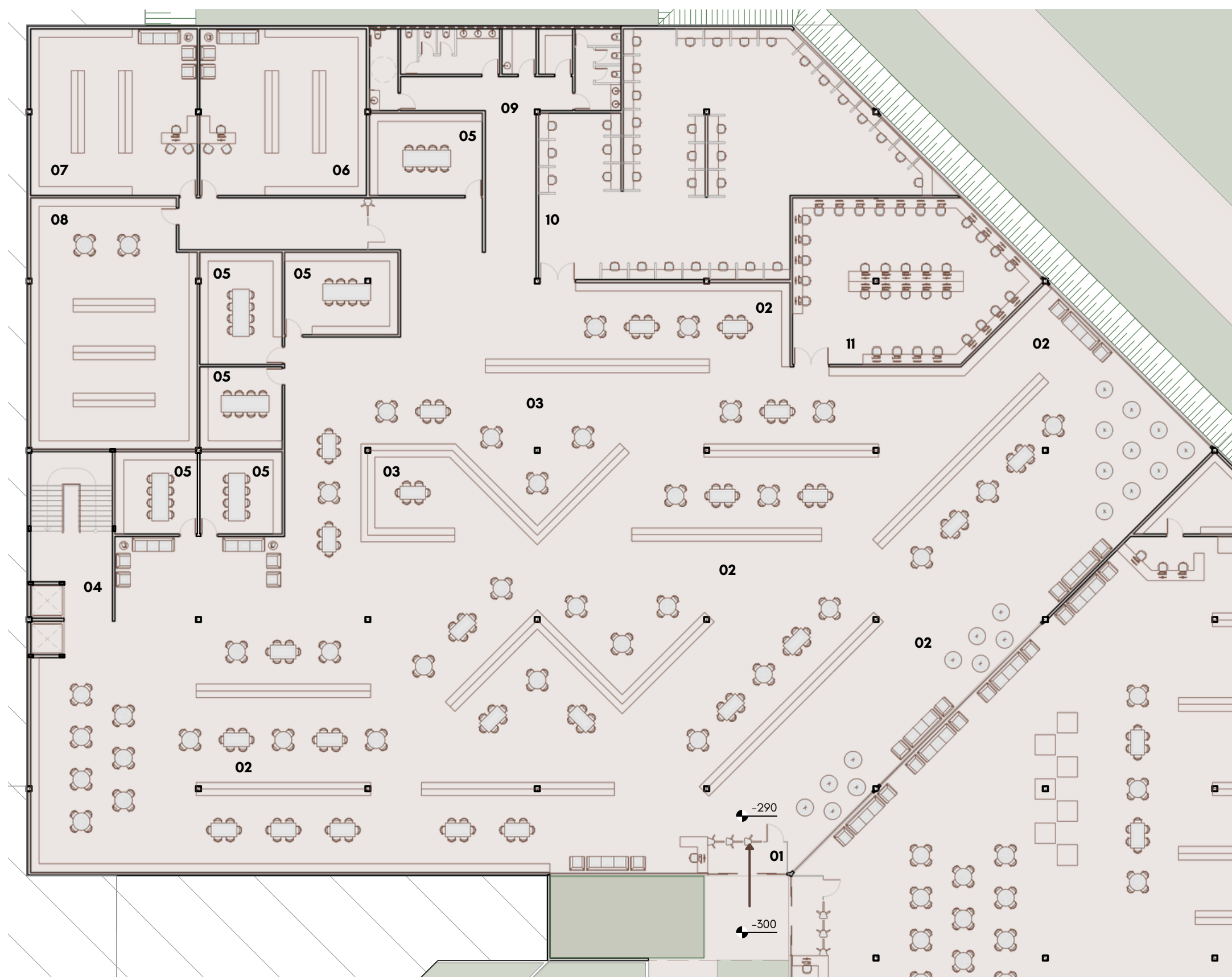
PLANTA DO SETOR DE ESTUDO E PESQUISA 0 1 5m
