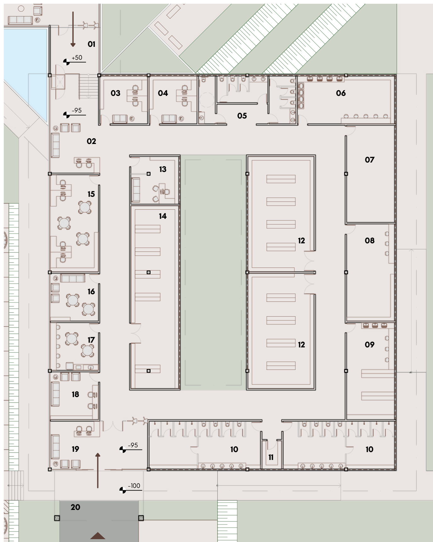
PLANTA DO SETOR ADMINISTRATIVO E DE SERVIÇOS
