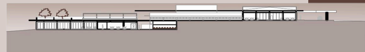
AMPLIAÇÃO CORTE CC 0 5 10 25m
