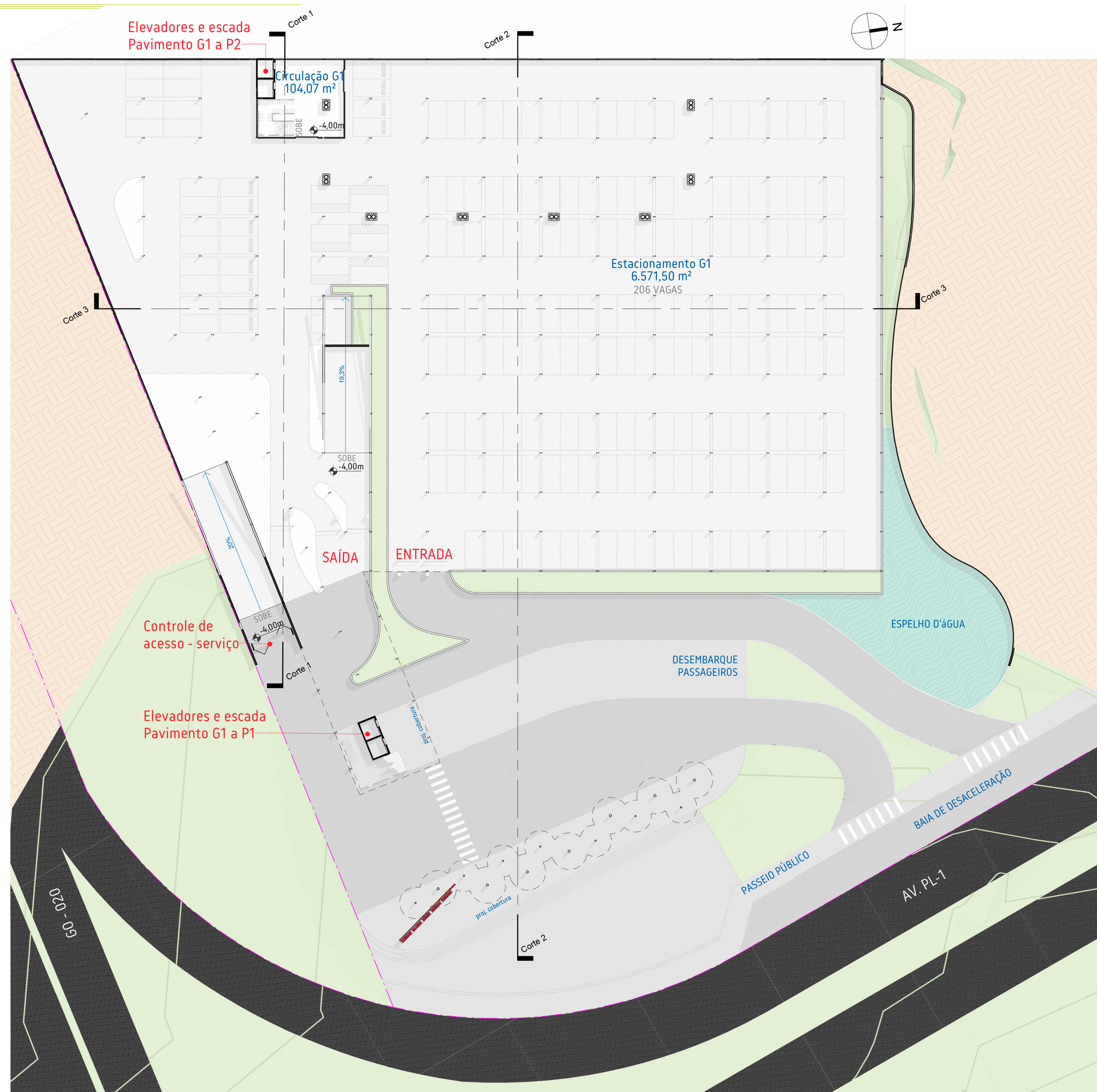
PLANTA DO PAV. G1 0 2 4 6 10 1:100
