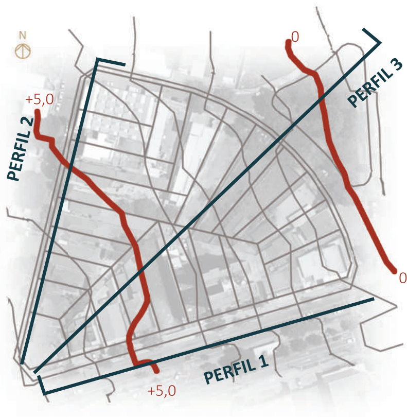
Figura 5.15 Levantamento Topográfico
