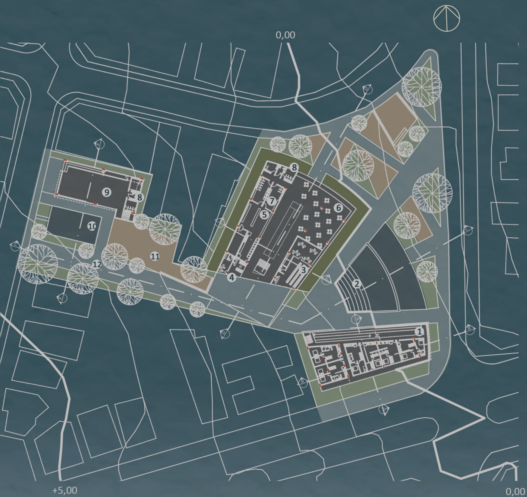
3 PLANTA TÉRREDO 2 - NÍVEL 1 0 5 15 1 10 30
