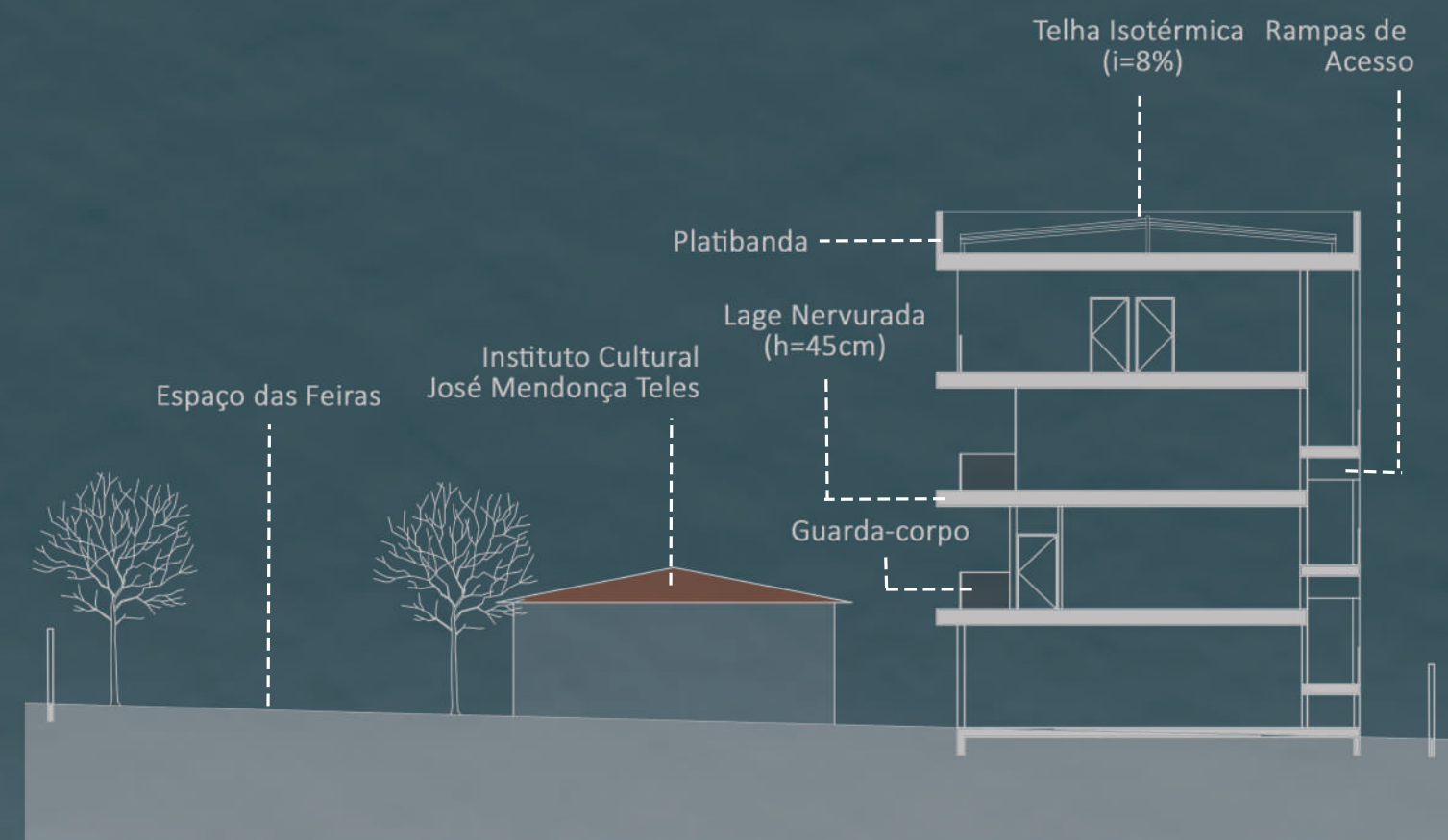
12 CORTE F 0 5 15 1 10
