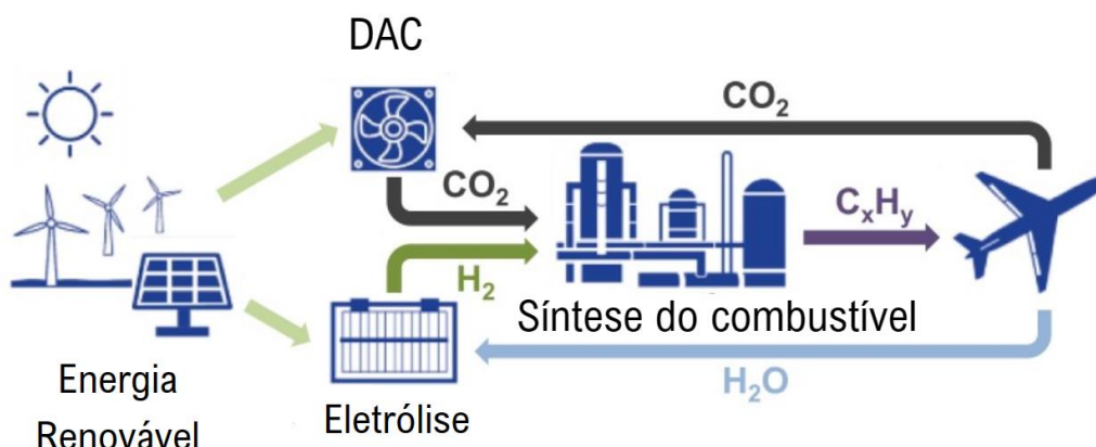
Figura 4: Esquema retratando a o processo PtL com o uso do DAC
