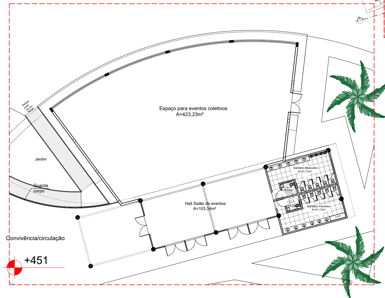
05 Planta Salão eventos +451
