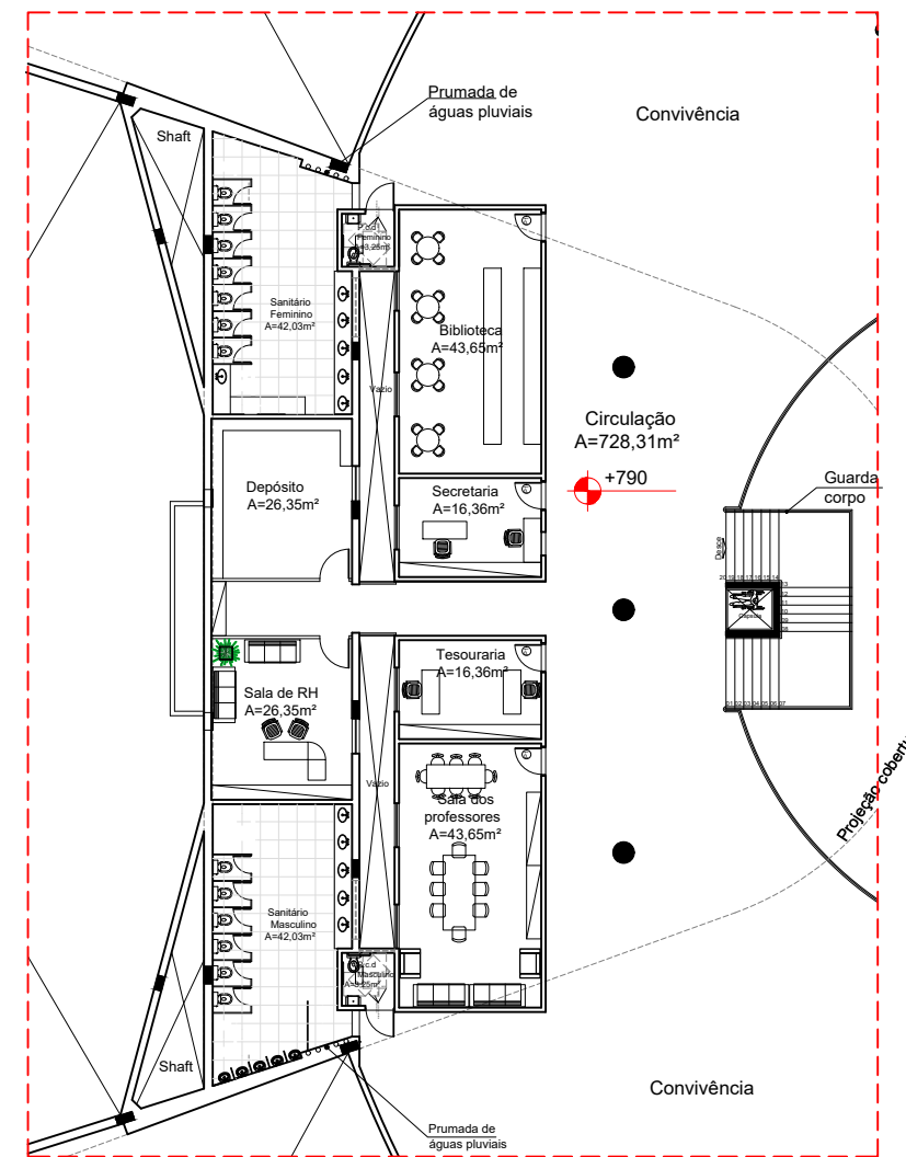
07 Planta Coordenação Escola Bíblica +790
