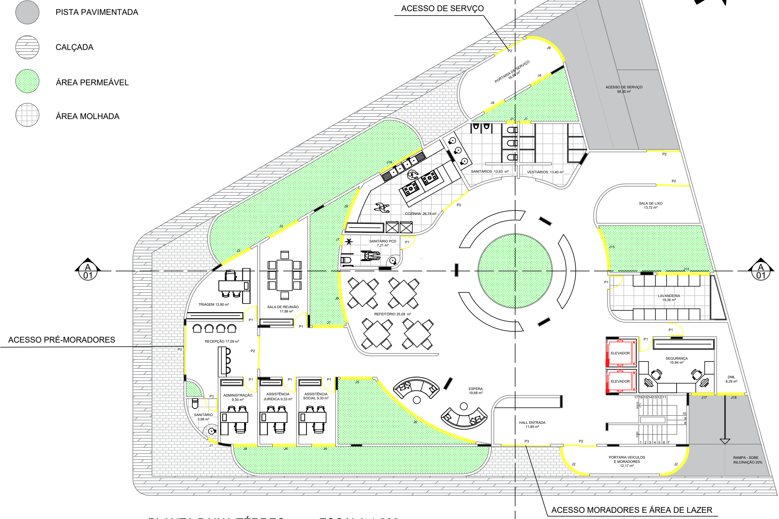
PLANTA BAIXA TÉRREO ESCALA 1:200
