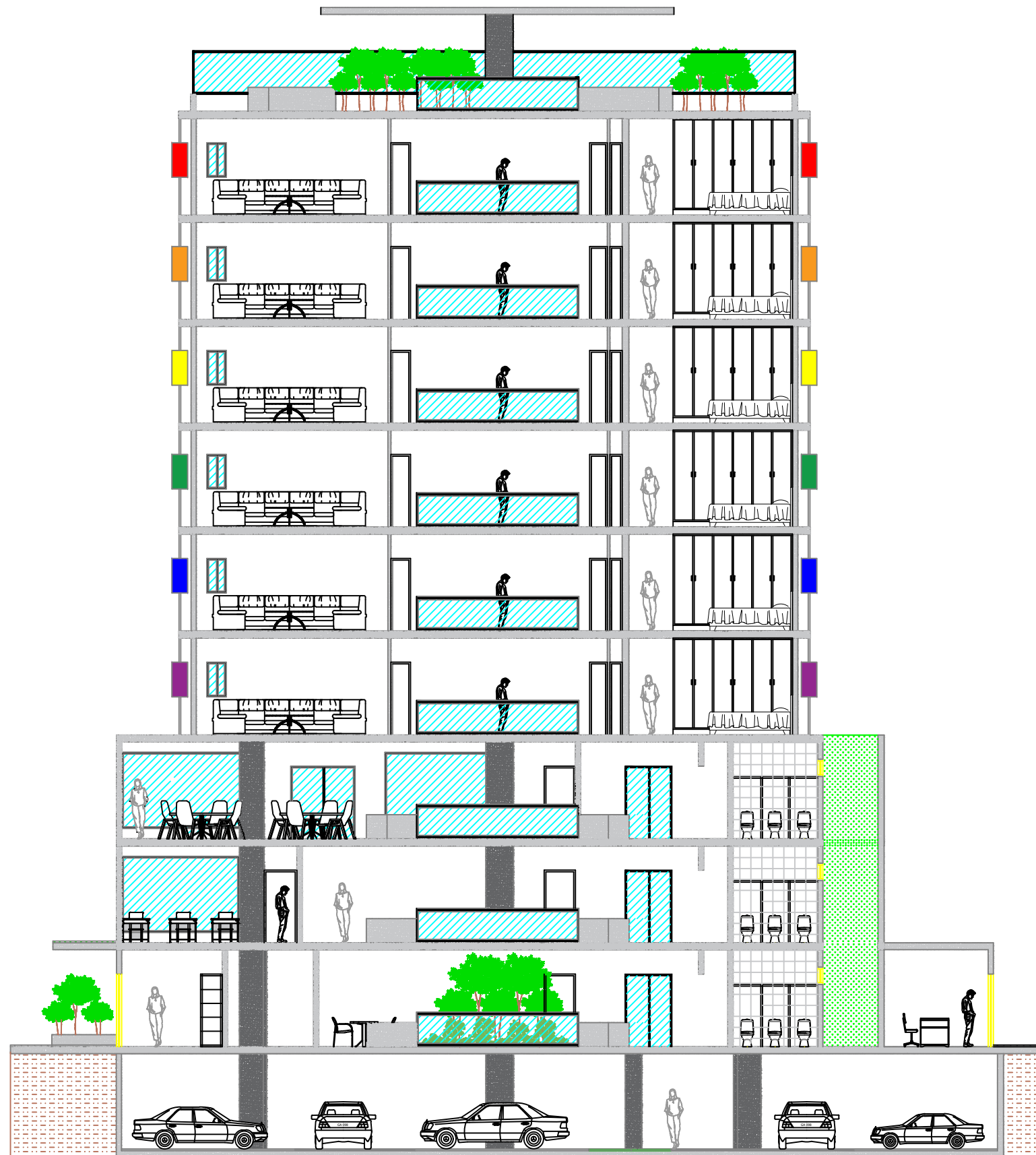
CORTE BB ESCALA 1:200
