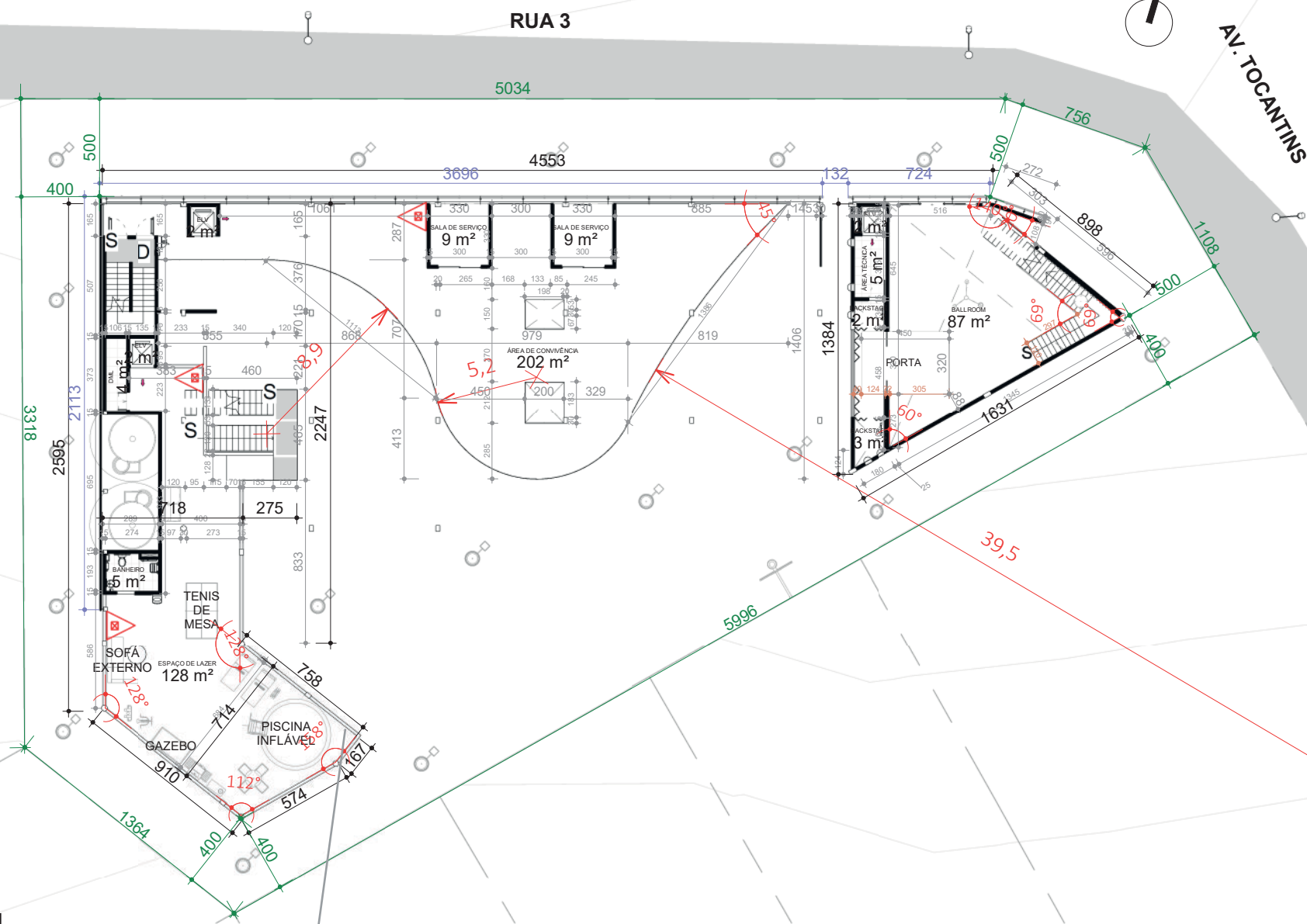
1 PAV 1 ESCALA 1 : 300
