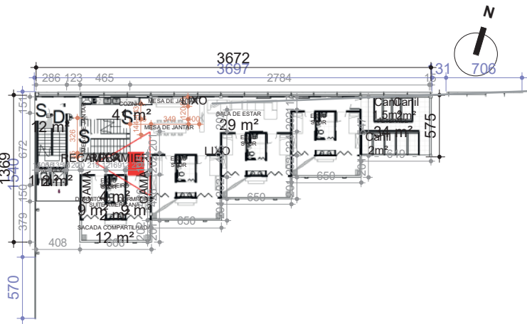
5 PAV 5 ESCALA 1 : 500
