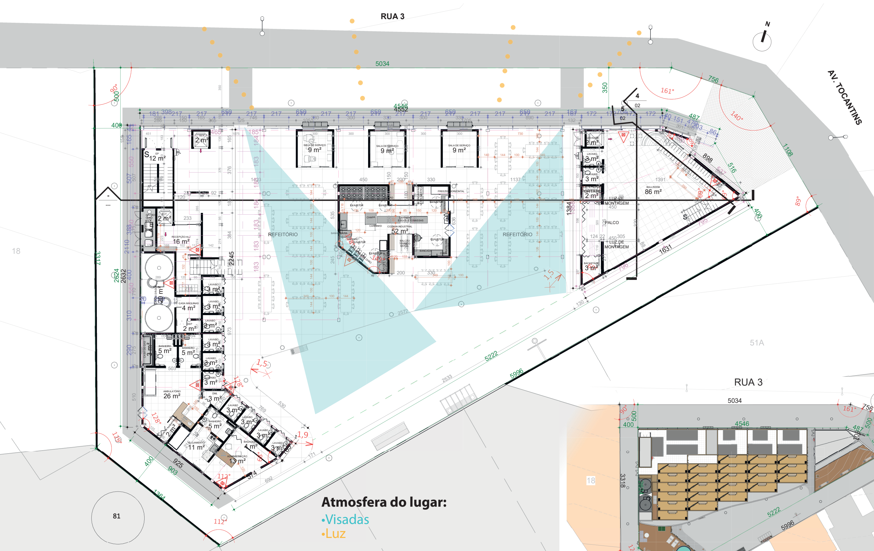
6 PLANTA TÉRREO ESCALA 1:200
