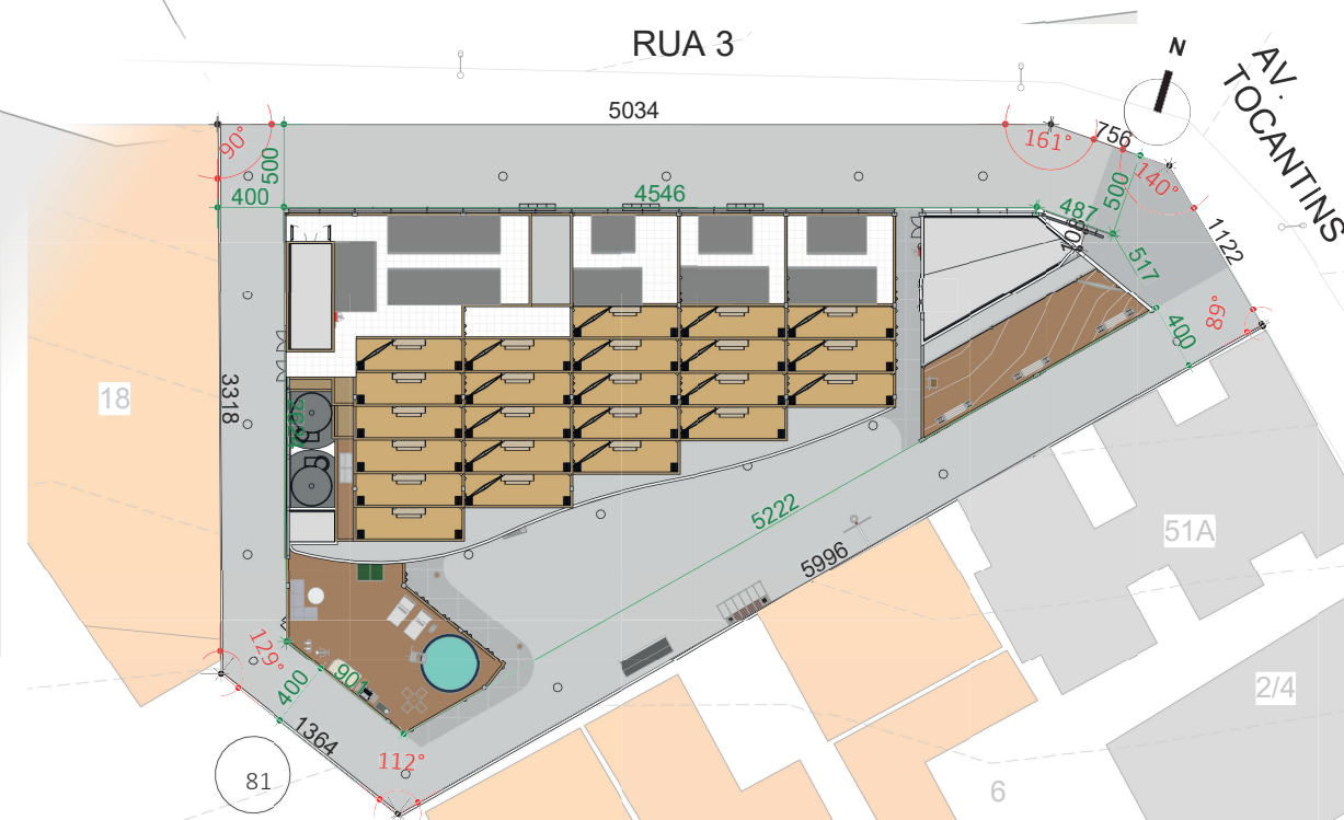
2 PLANTA IMPLANTAÇÃO ESCALA 1:500
