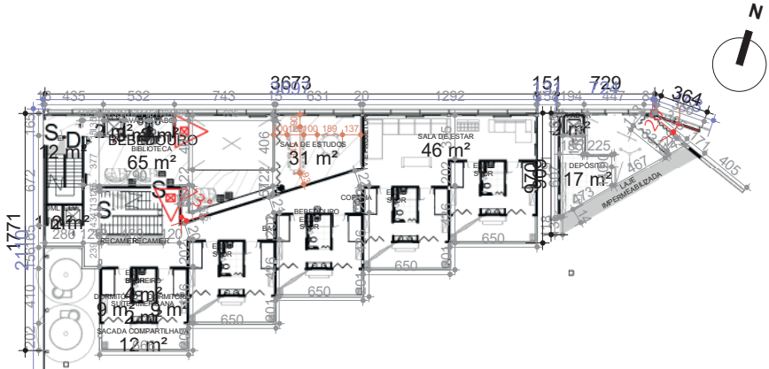
3 PAV 3 ESCALA 1 : 500
