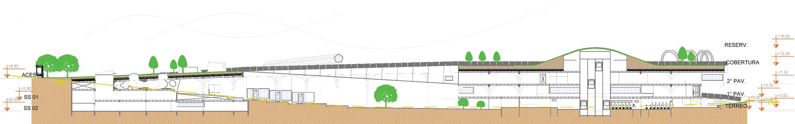
CORTE A
