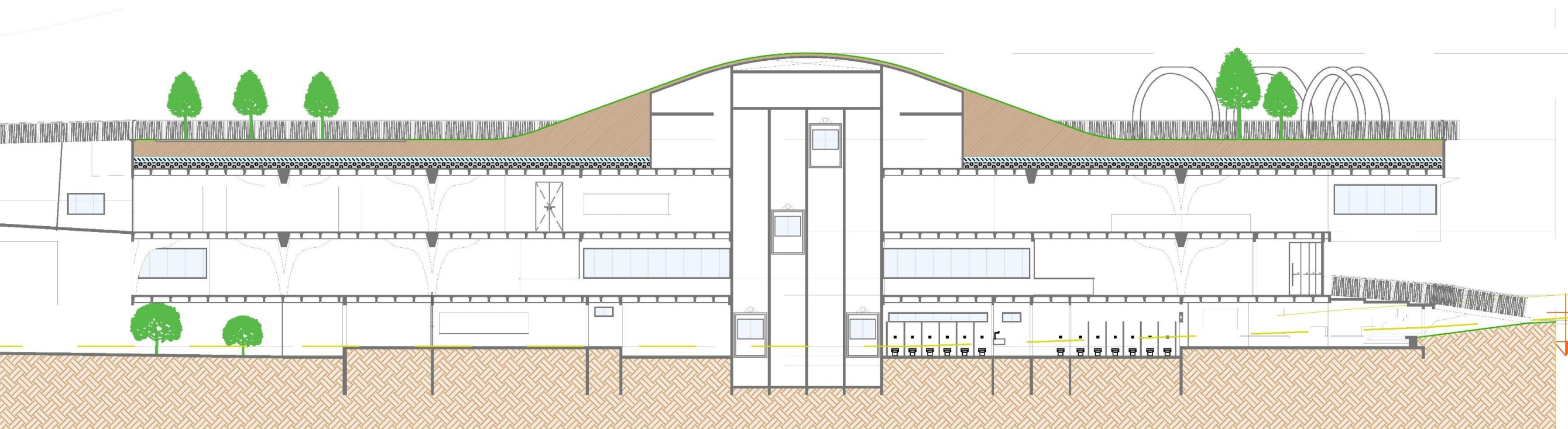
CORTE A
