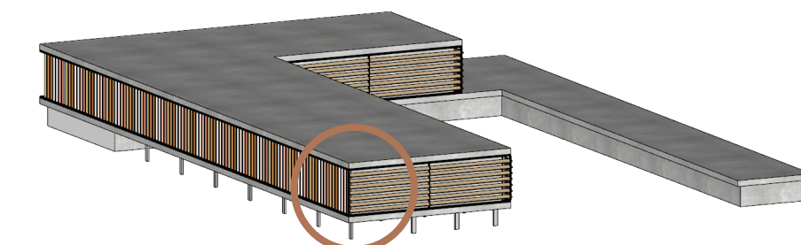
2 Brise horizontal fachada Nordeste e vertical fachada Sudoeste
