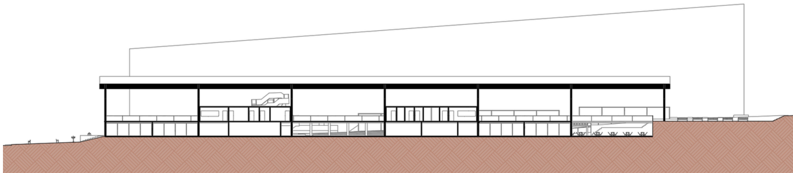
CORTE B
