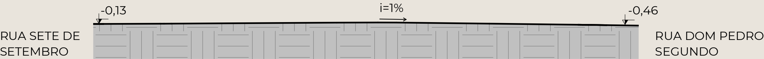
Corte A
